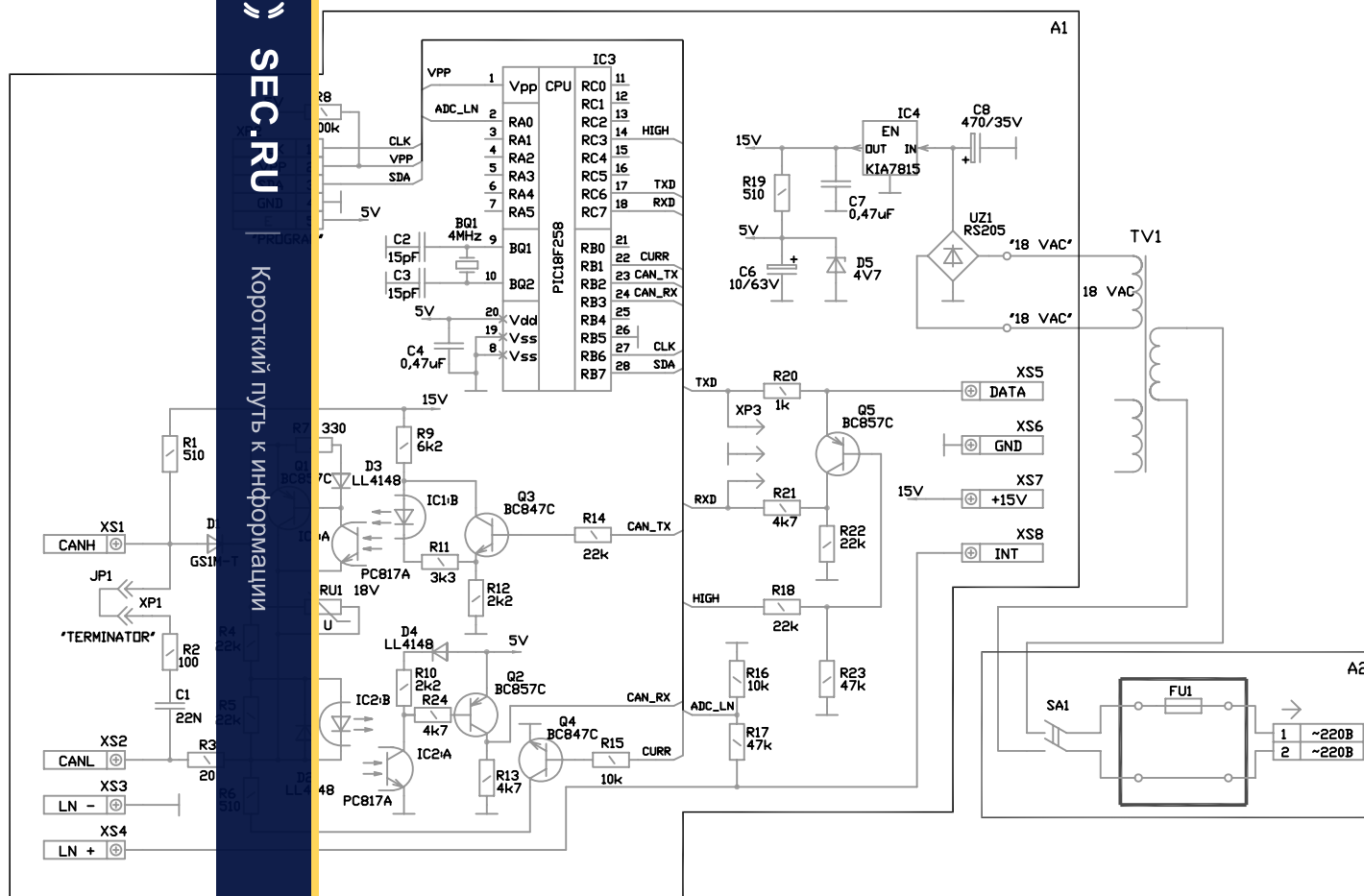
VIZIT-TU418 Схема электрическая принципиальная
