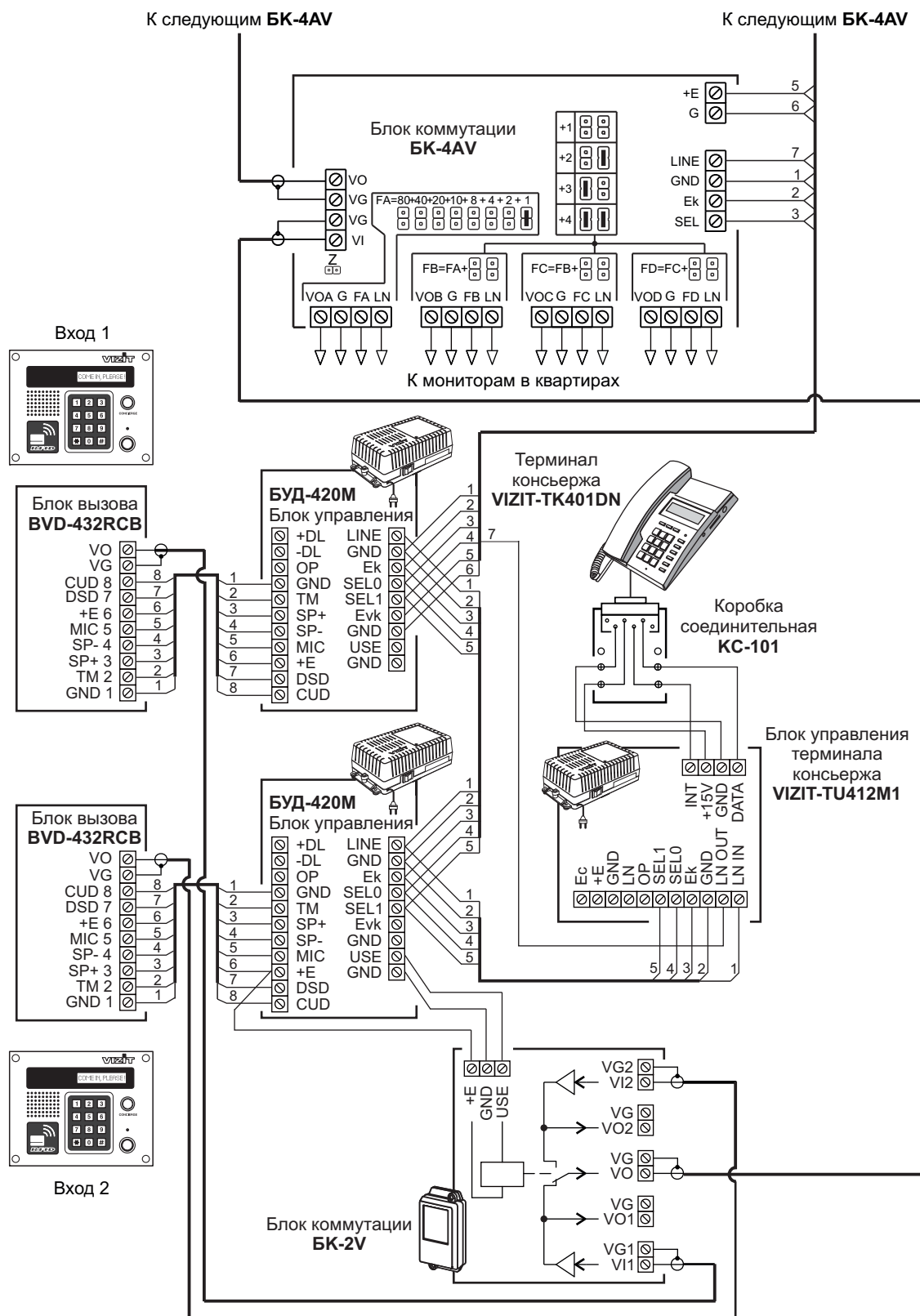
Рисунок 5 - Схема соединений пульта консьержа в составе 200-квартирного видеодомофона с двумя подъездными БВД
