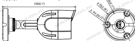
Рис.4 Габаритные размеры видекамеры
