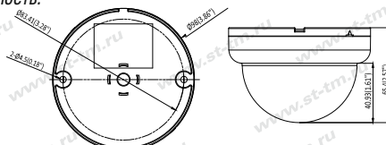
Рис.4 Габаритные размеры видекамеры
