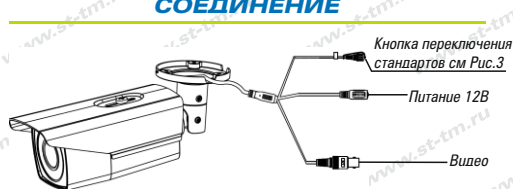
Рис.1 Схема подключения
