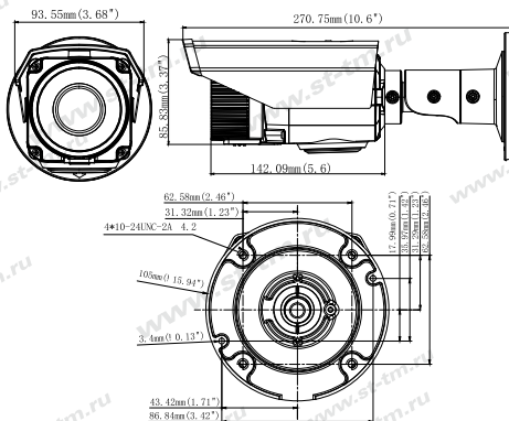
Рис.4 Габаритные размеры видеокмеры
