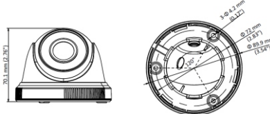
Рис.4 Габаритные размеры видекамеры
