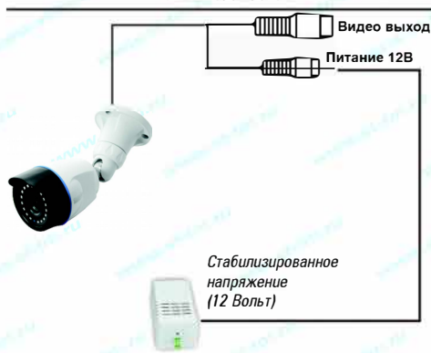
Рис.1 Схема подключения
