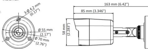
Рис.4 Габаритные размеры видекамеры
