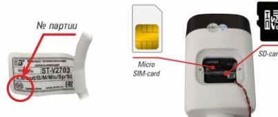
Схема №2 Вариант установки SIM-карты и карты памяти в камеру партии №98
