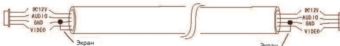
Экранированный кабель (≤ 80м)
