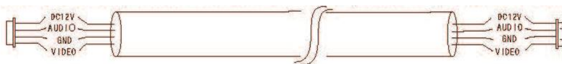
Неэкранированный кабель (≤ 50м)
