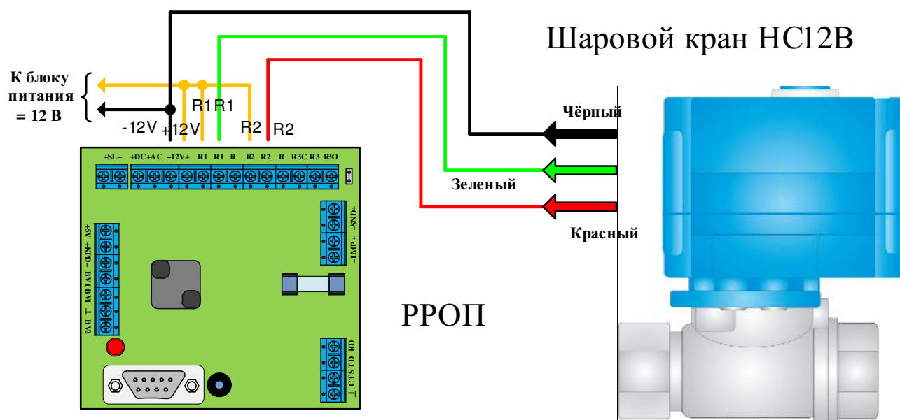
Рис. 6 Схема подключения крана HC12B к реле Р1 и Р2 РРОП.
