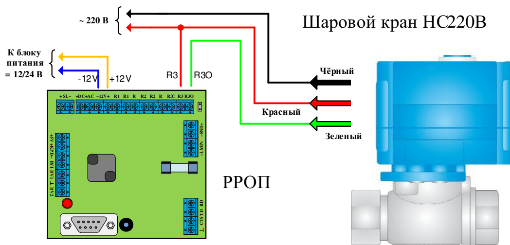
Рис. 10 Схема подключения крана HC220В к реле РРОП
