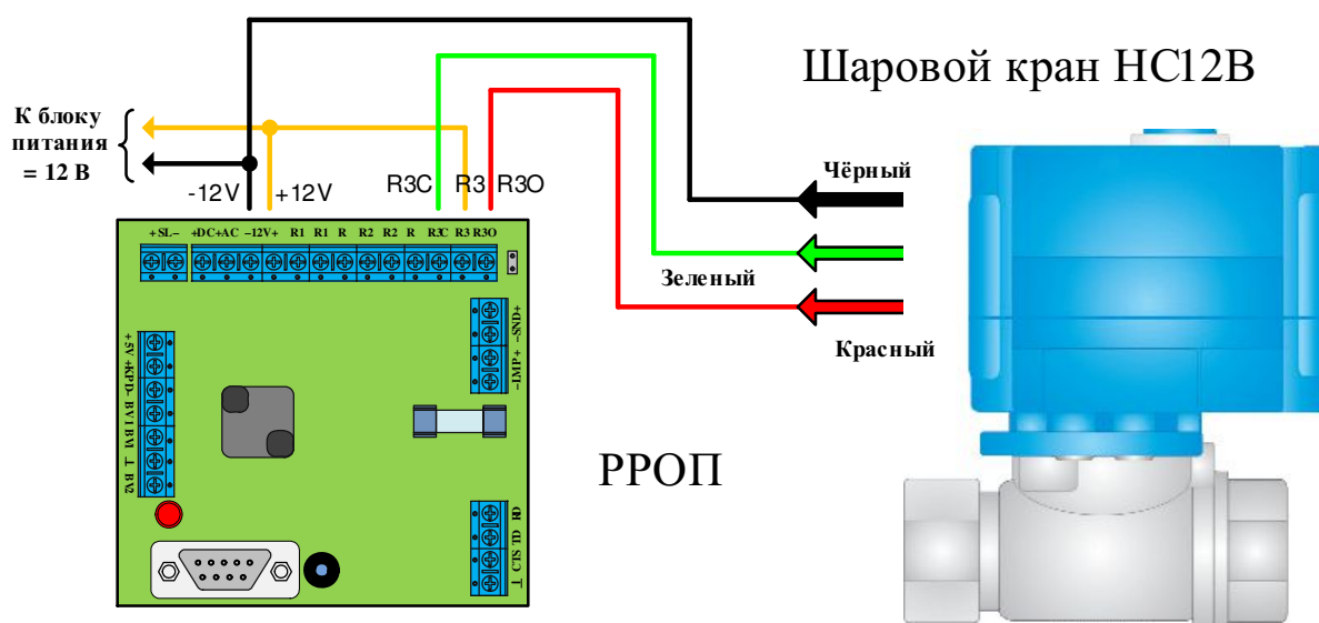
Рис. 5 Схема подключения крана HC12B к реле Р3 РРОП.
