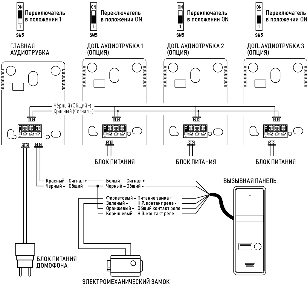
Рис.1 Схема подключения дополнительной аудиотрубку VOICE
