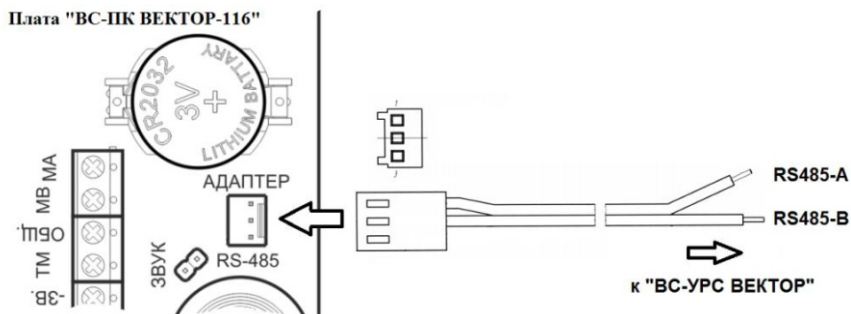
Рис 4. Схема оперативного временного подключения «BC-ПК ВЕКТОР-116» к «BC-УРС ВЕКТОР»
