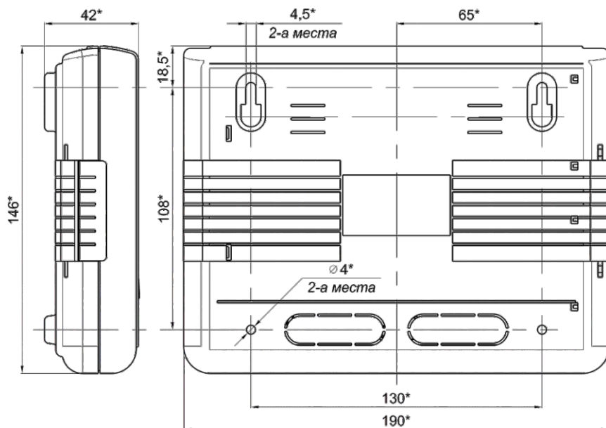
Рис 2. Габаритные и установочные размеры «BC-UPC BEKTOP»
