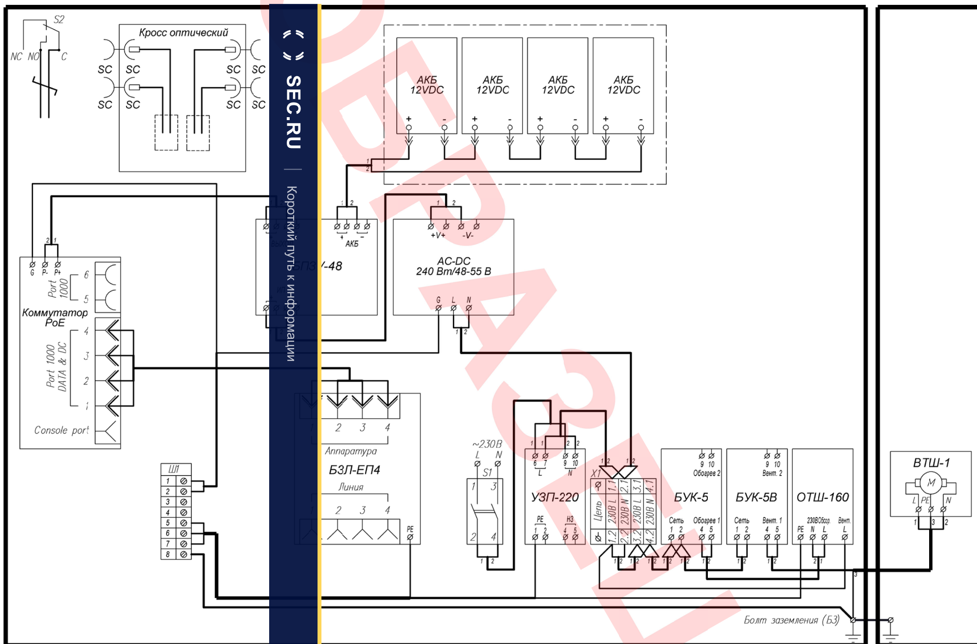
Рисунок 2 – Схема электрическая принципиальная
