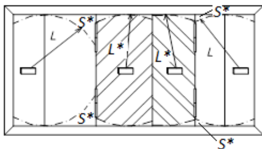
Рисунок 5. Защита немонолитной конструкции ( S^*<0,1\text{м}^2 , L<L^* )
