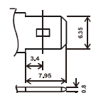
F2 (FASTON TAB 250)
