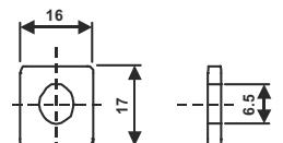
F4 (БОЛТ И ГАЙКА M6)
