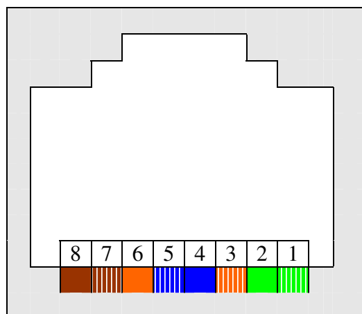
Рис. 3. Нумерация контактов
