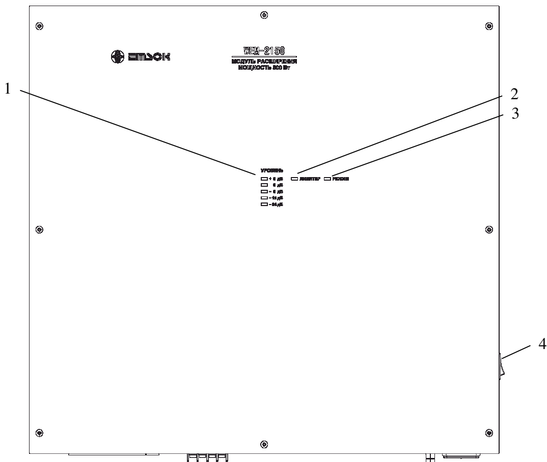
Рис. 1. Передняя панель модуля расширения. 1 – индикатор уровня выходного сигнала, 2 – индикатор срабатывания лимитера, 3 – индикатор режима работы, 4 – выключатель сетевого питания.
