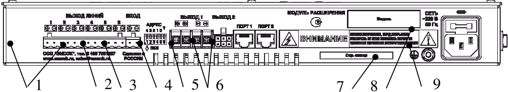
Рис. 2. Нижняя панель модуля расширения. 1 – выход линий (коммутируемый), 2 – резервный вход коммутатора, 3 – переключатель адреса, 4, 5 – некоммутируемые выходы модуля расширения, 6 – порт связи, 7 – клемма защитного заземления, 8 – сетевой предохранитель, 9 – соединитель сетевого питания.
