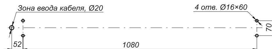
Разметка отверстий для монтажа калитки
