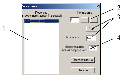
Рисунок 7.13. Диалоговое окно конфигурирования усилителей. 1 – перечень усилителей, 2 – элементы управления количеством усилителей, 3 – настройки каждого усилителя, 4 – общие параметры усилителей.
