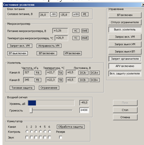
Рисунок 7.48. Окно просмотра состояния и управления усилителем.
