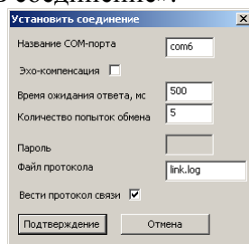
Рисунок 7.56. Диалоговое окно установки связи.
