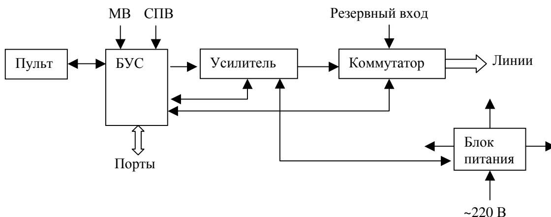
Рисунок 6.3. Структурная схема станции.
