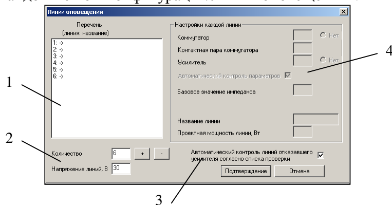
Рисунок 7.16. Диалоговое окно конфигурирования линий оповещения. 1 – перечень линий оповещения, 2 – элементы управления количеством, 3 – поле ввода номинального напряжения линий, 4 – параметры каждой линии.
