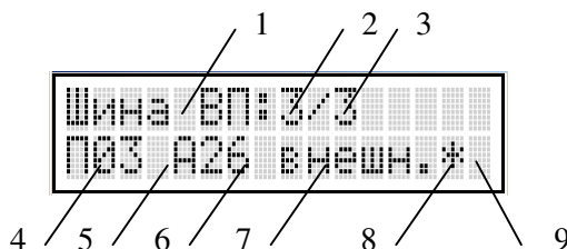
Рисунок 8.43. Экран в режиме описания подключения внешних устройств. 1 – тип устройства, 2 – порядковый номер устройства, 3 – количество устройств заданного типа, 5 – номер порта, 6 – символ неправильно выбранного порта для заданного типа устройства, 7 – адрес, 8 – расположение, 9 – режим питания, 10 – подтип устройства.
