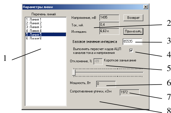
Рисунок 7.53. Диалоговое окно измерения параметров линий. 1 – перечень линий оповещения, 2 – измеренные значения (напряжение, ток, импеданс), 3 – эталонное значение импеданса, 4 – переключатель пересчета кодов АЦП, 5 – результаты сравнения, 6 – примерная мощность линии, 7 – измеренное значение утечки, 8 – информационная строка.
