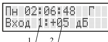
Рисунок 8.10. Основной экран в режиме отображения добавочной громкости. 1 – Номер линейного входа, 2 – добавочная величина.
