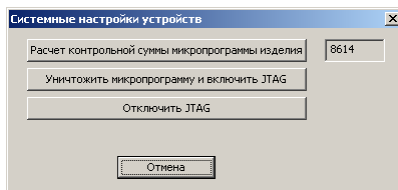
Рисунок 7.51. Окно просмотра состояния и управления усилителем.
