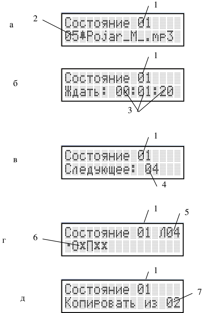
Рисунок 8.38. Экран в режиме редактирования пожарного состояния. а – страница установки файла, б – страница установки времени ожидания, в – страница установки следующего состояния,
