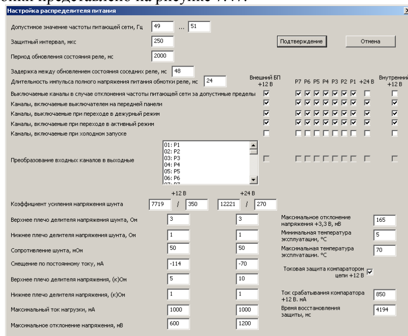
Рисунок 7.47. Окно редактора конфигурации распределителя питания.
