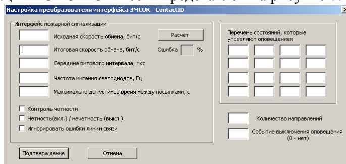
Рисунок 7.41. Окно редактора конфигурации БСПС «Юнитест».
