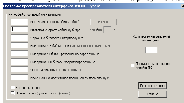
Рисунок 7.39. Окно редактора конфигурации БСПС «Рубеж».
