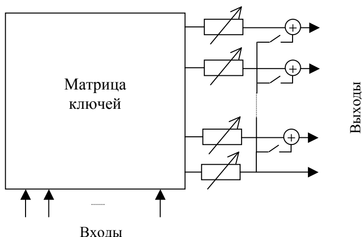
Рисунок 6.5. Схема прохождения сигнала через аналоговую матрицу.
