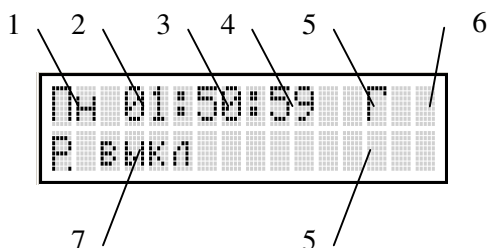
Рисунок 8.9. Основной экран в режиме отображения состояния. 1 – День недели, 2 – час, 3 – минута, 4 – секунда, 5 – состояния виртуальных источников, 6 – символ оповещения, 7 – название текущего расписания.
