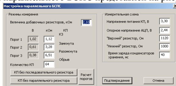
Рисунок 7.37. Окно редактора настроек параллельного БСПС.
