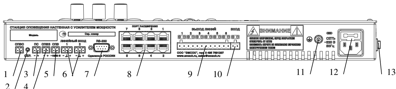
Рисунок 6.2. Нижняя стенка станции. 1 – Выход подтверждения включения трансляции сигнала СПВ, 2 – кнопка перезагрузки, 3 – вход запуска НПО «1», 4 – вход запроса включения трансляции СПВ, 5 – вход сигнала СПВ, 6 – входы МВ, 7 – порт RS-232, 8 – порты 1-8, 9 – выход линий оповещения, 10 – вход для резервного усилителя, 11 – клемма заземления, 12 – соединитель подачи питания с держателем плавкой вставки, 13 – выключатель питания.
