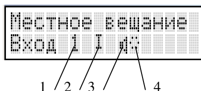
Рисунок 8.17. Экран в режиме включения/выключения местного вещания. 1 – номер входа, 2 – 2 – символ действия оператора, 3 - символ наличия сигнала, 4 – символ выполнения выдержки перед отключением.
