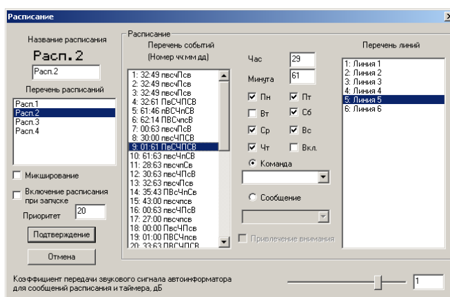
Рисунок 7.24. Диалоговое окно конфигурирования расписания.
