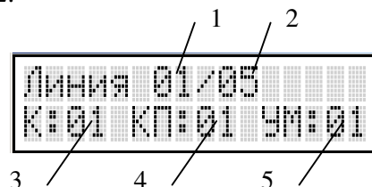
Рисунок 8.42. Экран в режиме задания параметров линий оповещения. 1 – Номер текущей линии, 2 – количество линий, 3 – номер коммутатора текущей линии, 4 – номер контактной пары коммутатора текущей линии, 5 – номер усилителя текущей линии.
