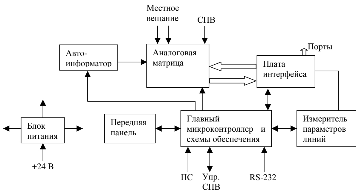
Рисунок 6.4. Структурная схема БУС.
