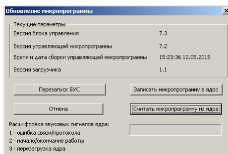
Рисунок 7.52. Диалоговое окно обновления микропрограммы главного микроконтроллера станции.
