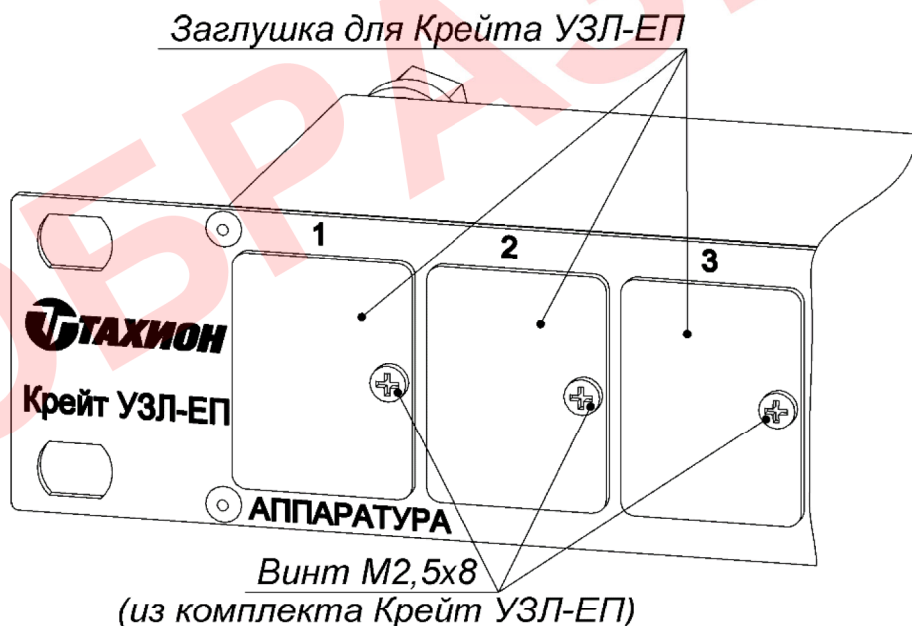
Рисунок 1 – Установка изделия
