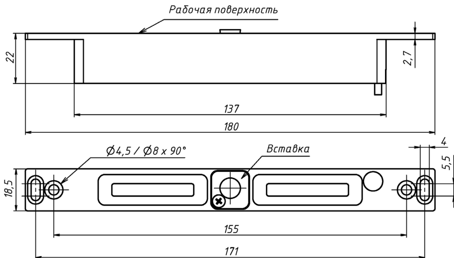
Рисунок 6 – Корпусная часть замка AL-250SM
