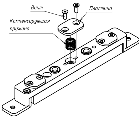
Рисунок 4 – Демонтаж пружины якоря для вертикального варианта замка
