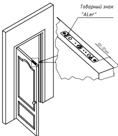
Рисунок 3 – Установка замка в горизонтальном варианте
