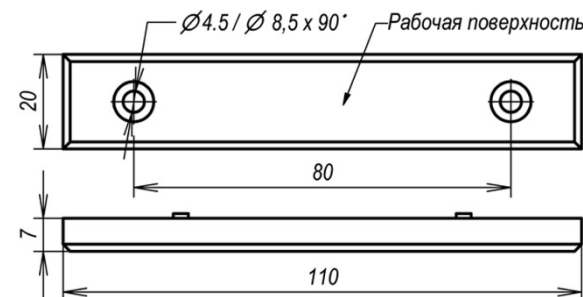
Рисунок 3 – Якорь
