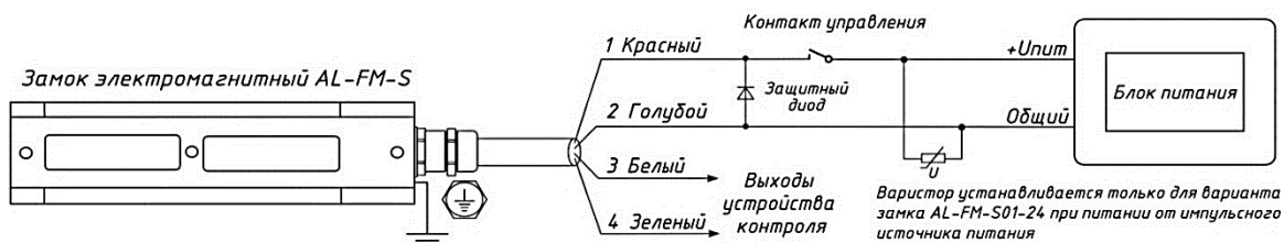
Рисунок 9 - Схема подключения изделия для вариантов «Н» и «Г»
