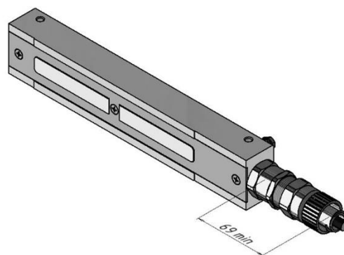
Рисунок 3 – Изделие варианта «М» базовой комплектации с кабельным вводом для присоединения металлорукава типа МРПИ 15
