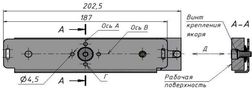
Рисунок 8 - Якорная часть замка варианта «Г»
