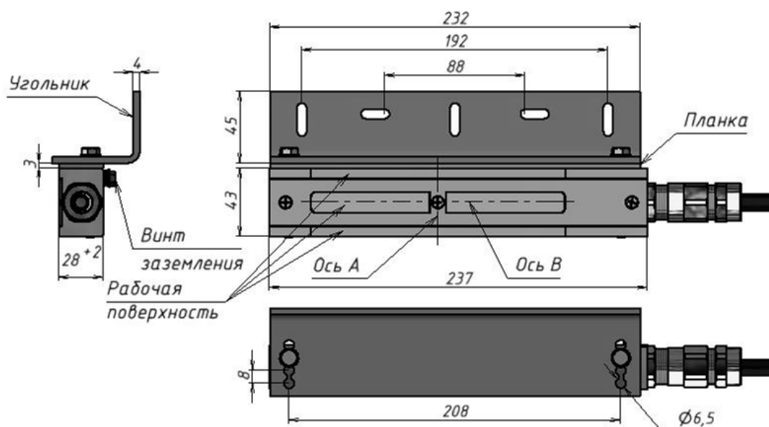
Рисунок 6 - Корпусная часть
