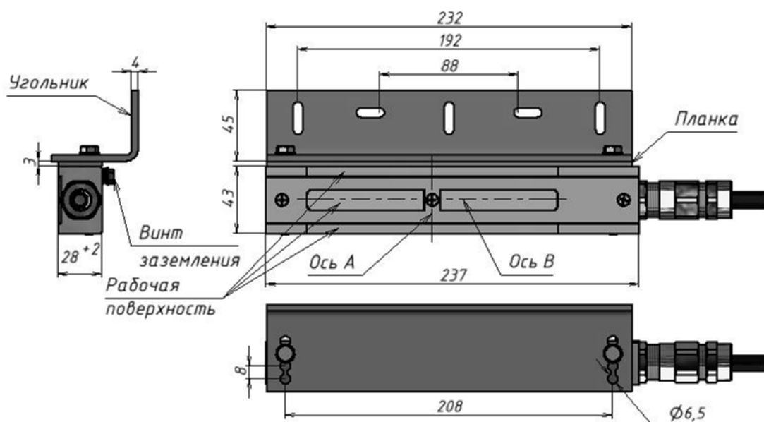
Рисунок 6 - Корпусная часть
