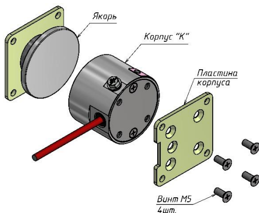
Рисунок 1 – Комплект поставки
