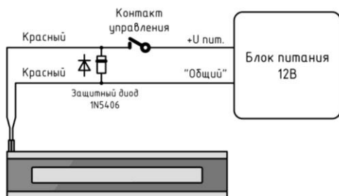
Рисунок 4 – Схема включения замка SEC.RU/ALM-180FB-12V
