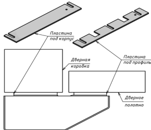
Рисунок 2 – Установка выравнивающих пластин под корпус и якорь
