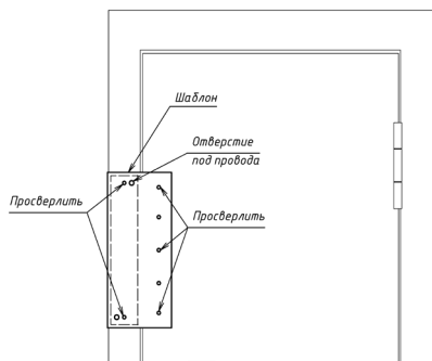
Рисунок 3 – Установка замка по шаблону
