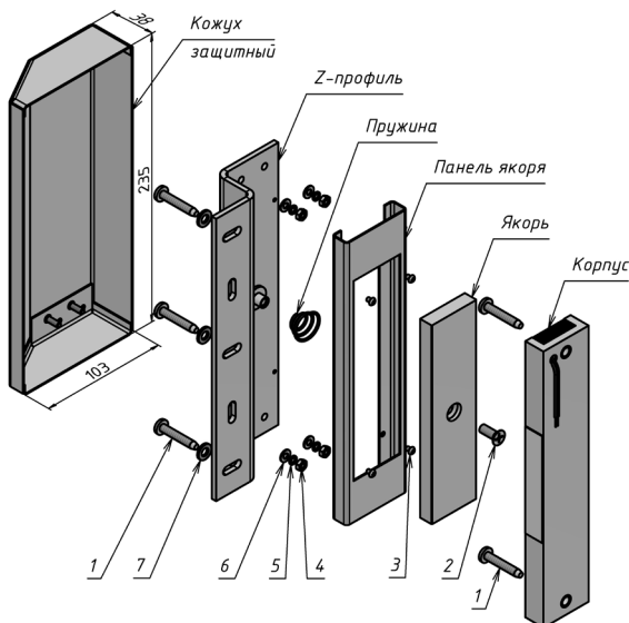
Рисунок 1 – Комплект поставки замка ALM-250FT-12/24V
