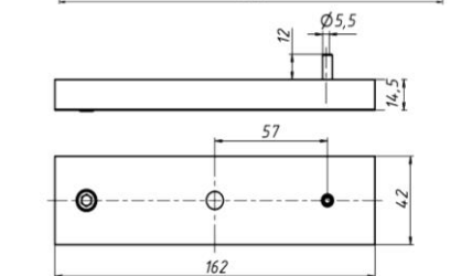
Рисунок 4 - Габариты якоря
