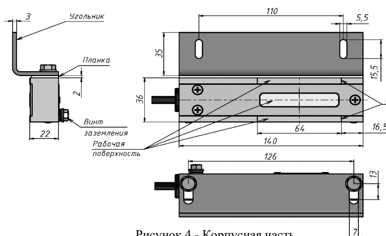
Рисунок 4 - Корпусная часть
