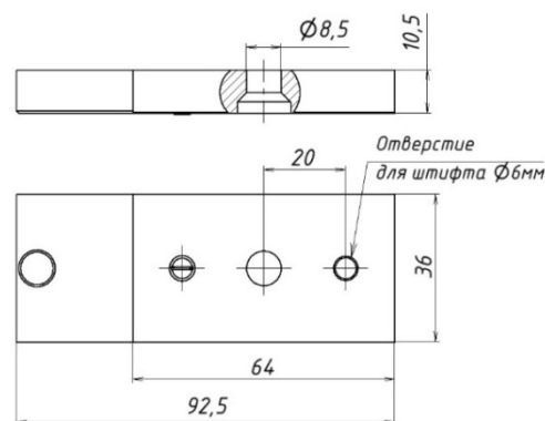
Рисунок 5- Габаритный чертеж якоря
