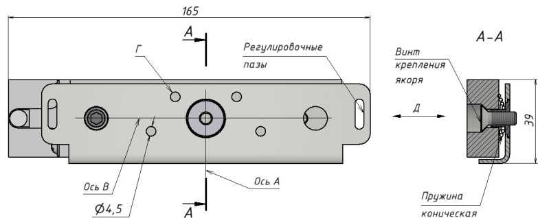
Рисунок 8 - Якорная часть замка варианта «Г»
