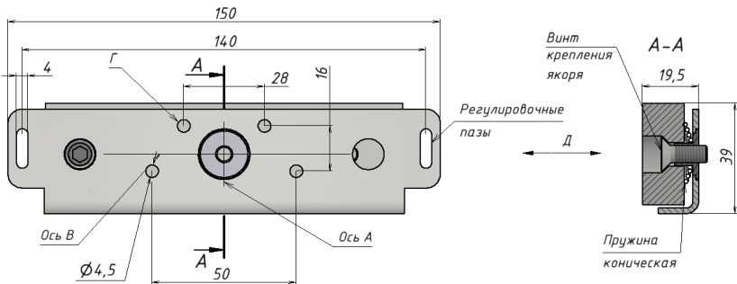
Рисунок 7- Якорная часть замка варианта
