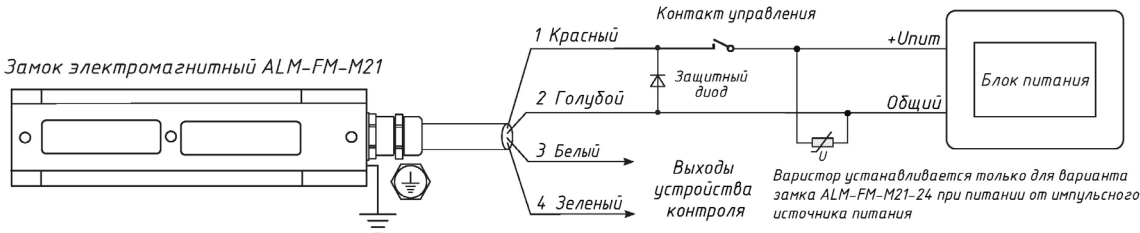
Рисунок 9 - Схема подключения изделия для вариантов «H» и «G»
