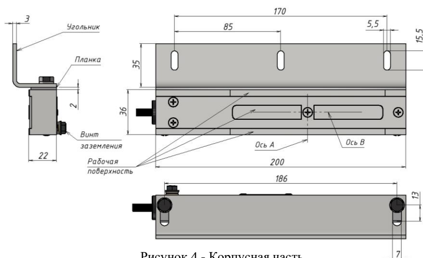
Рисунок 4 - Корпусная часть
