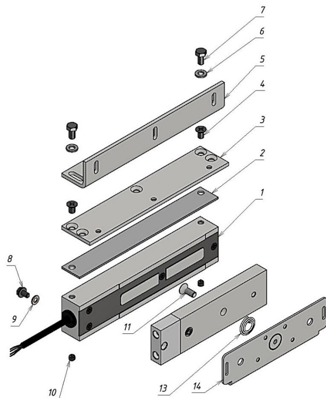
Рисунок 1 – Комплект поставки
