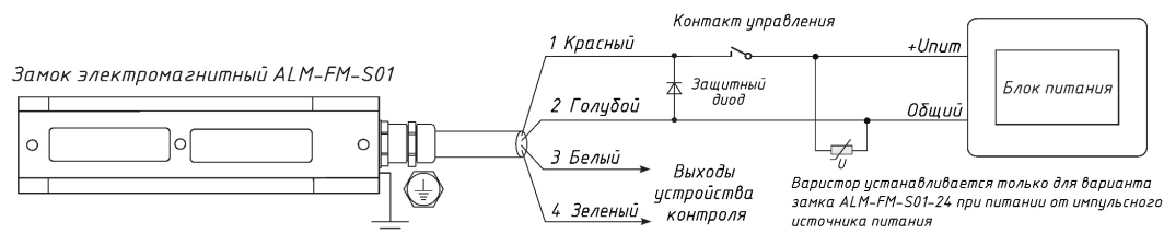
Замок электромагнитный ALM-FM-S01 1 Красный 3 Белый 2 Голубой 4 Зеленый Контакт управления Защитный диод +U пит Общий Блок питания Варистор устанавливается только для варианта замка АЛМ-FM-S01-24 при питании от импульсного источника питания
