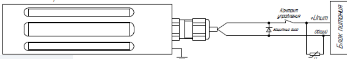
Замок электромагнитный Ex-замок FM-26
