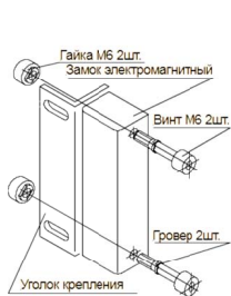
Рис. 1. Вариант крепления электромагнитного замка к раме двери.
