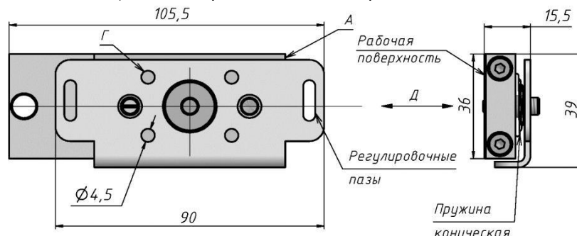
Рисунок 8 - Якорная часть замка варианта «G»
