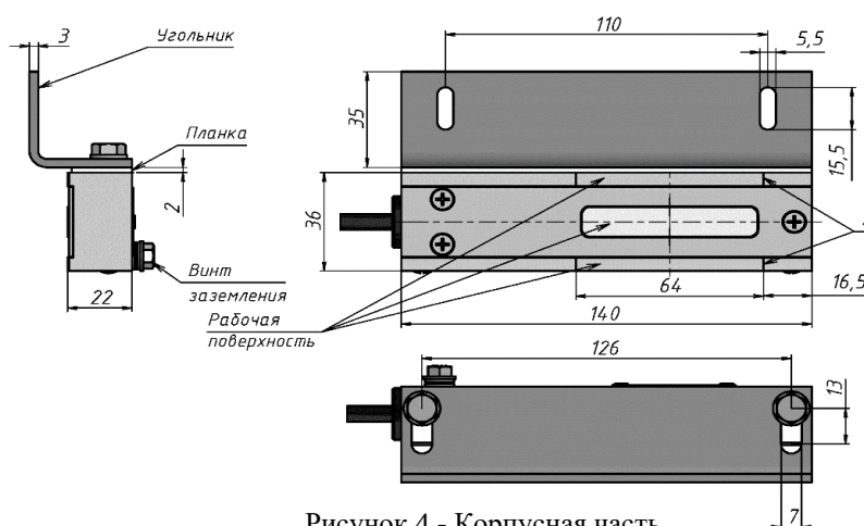
Рисунок 4 - Корпусная часть
