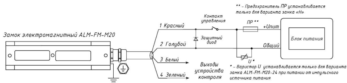
Рисунок 9 - Схема подключения изделия для вариантов «Н» и «Г»
