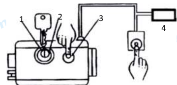
Рис.1. Части управления замка
