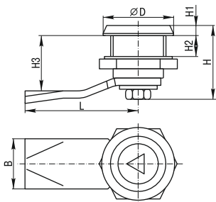
Рисунок 4. Замок-защёлка с трёхгранным ключом IP54 22-25/44
