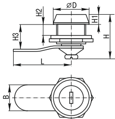
Рисунок 2. Замок 18-18/34
