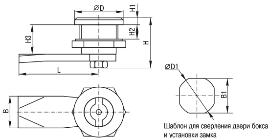
Рисунок 5. Замок-защёлка с пластмассовым ключом IP54 22-17/46
