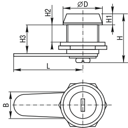
Рисунок 3. Замок 18-20/40
