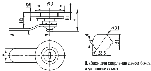
Рисунок 1. Замки 20-22/40, 20-22/45
