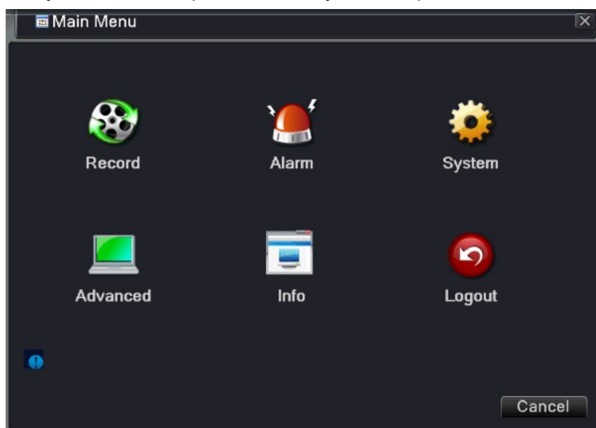
Рис. 3.3 Главное меню
