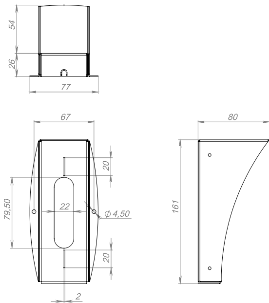
Рис. 1 Габаритные и установочные размеры
