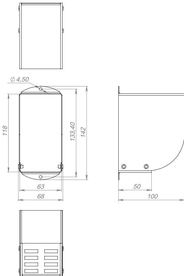
Рис. 1 Габаритные и установочные размеры
