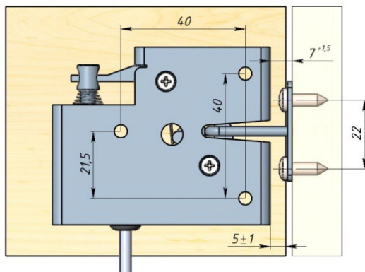
Присоединительные размеры корпусной части
