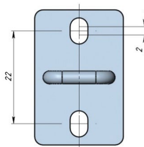
Присоединительные размеры зацепа
