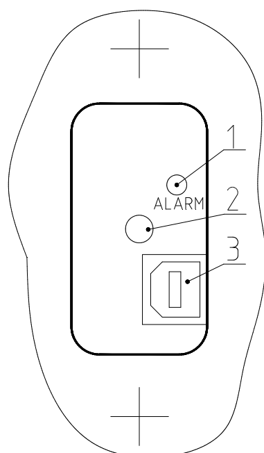
Рисунок 1.3 – Органы настройки блока ПРМ-ПРД извещателей «ЗЕБРА-60(24)»
